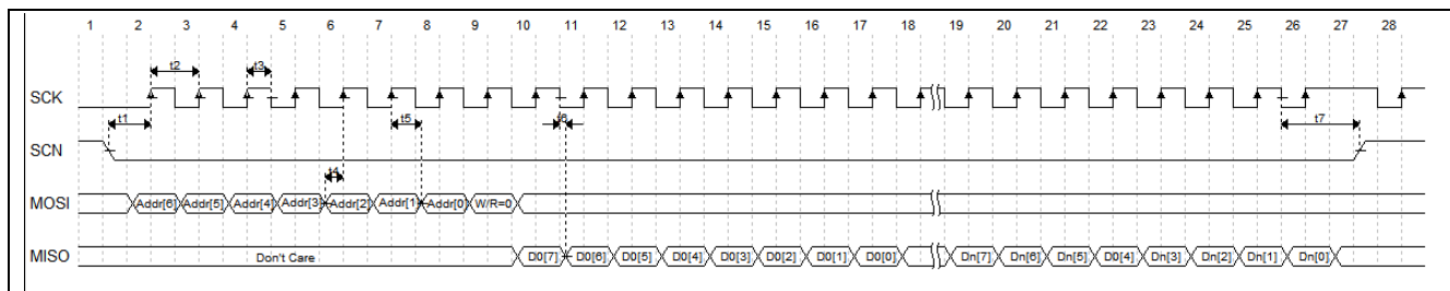
图 9-2 SPI 读时序
