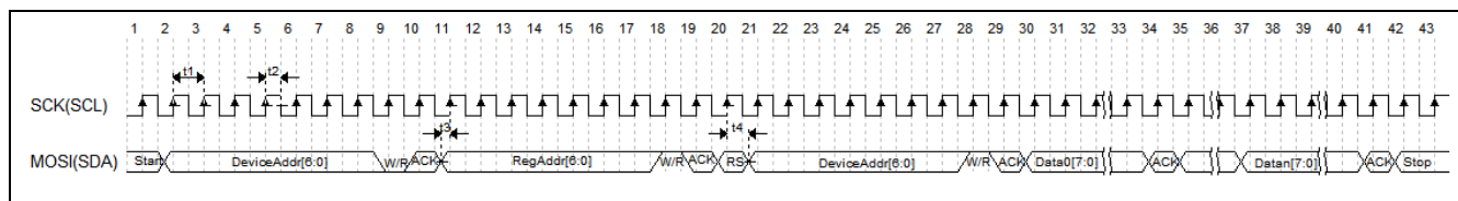
图 9-8 I2C 读时序
