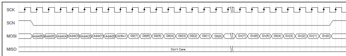
图 9-1 SPI 写时序
